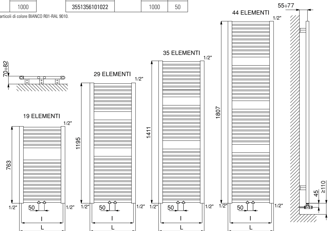
Particolare della versione Interasse 50 mm.
