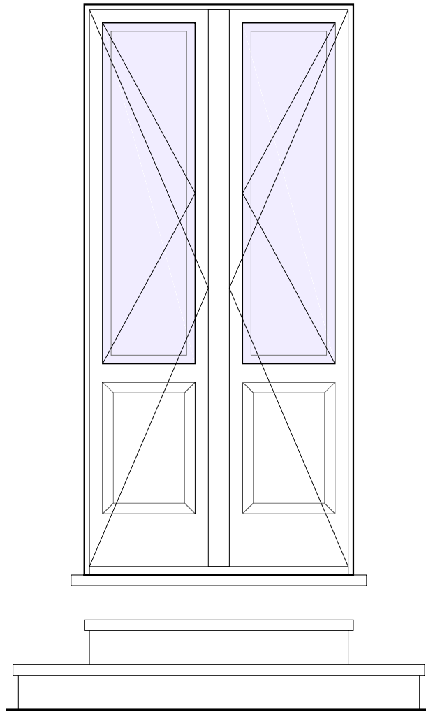
se.26 portafinestra scala piano primo dim. vano luce cm 102x216h superficie mq 2.20 movimento apertura alla francese vetri 3+3/16/3+3 trasparente scuri interni
