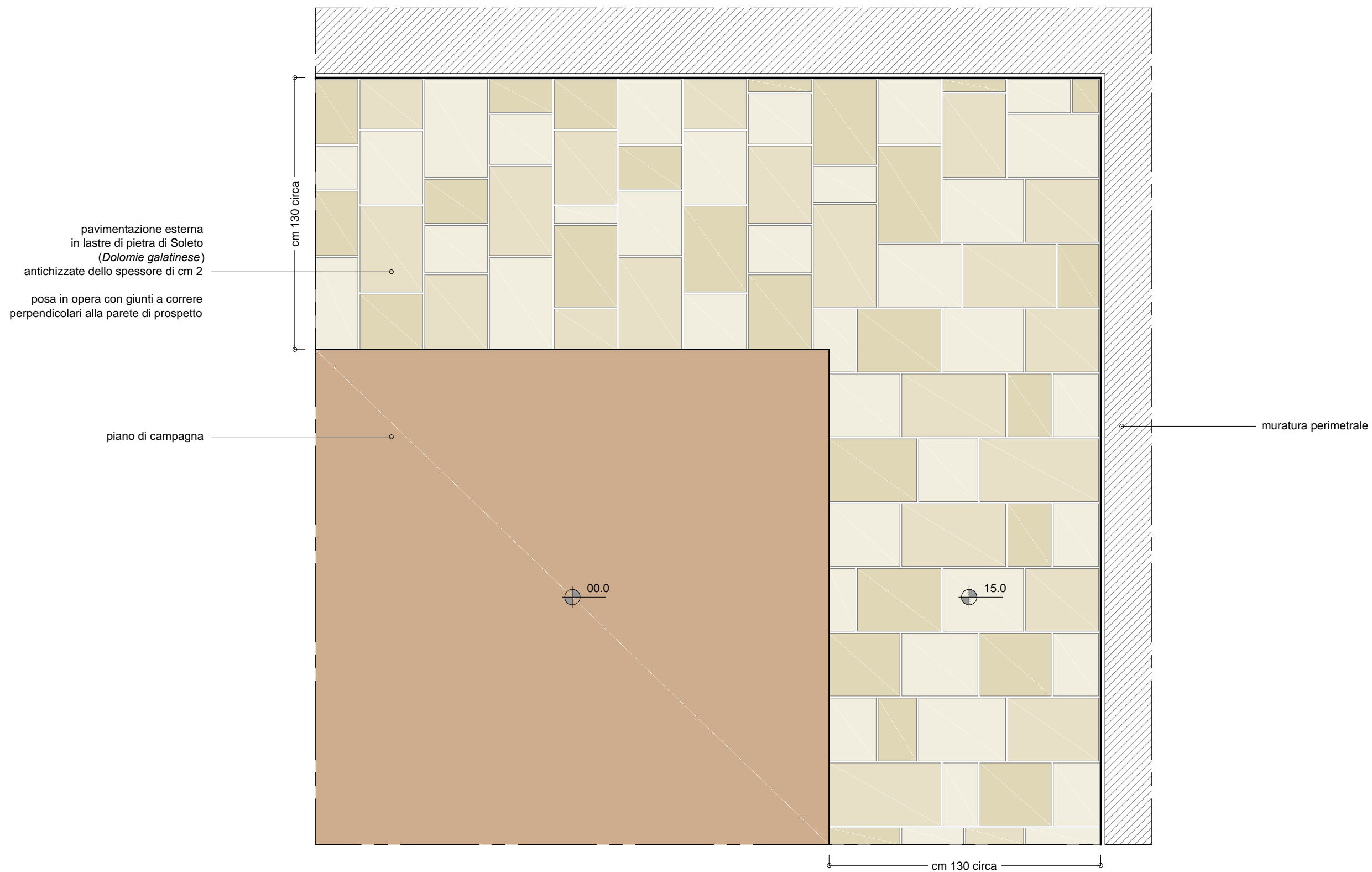
B SCHEMA DI POSA NELLE SOLUZIONI D'ANGOLO
