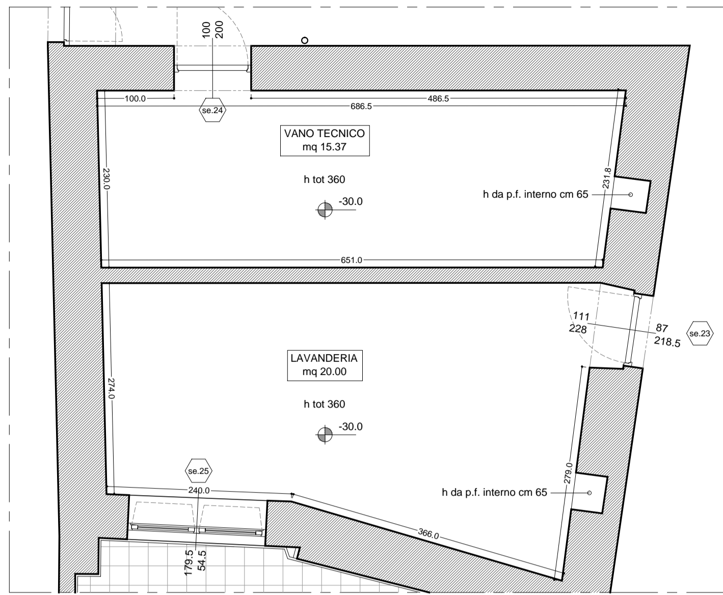
PIANO TERRA - ala est
